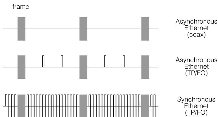
Obrázek 8.11: Synchronní Ethernet
