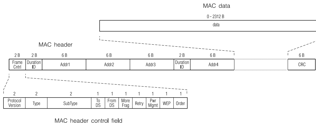
Obrázek 13.10: Formát rámců MAC
