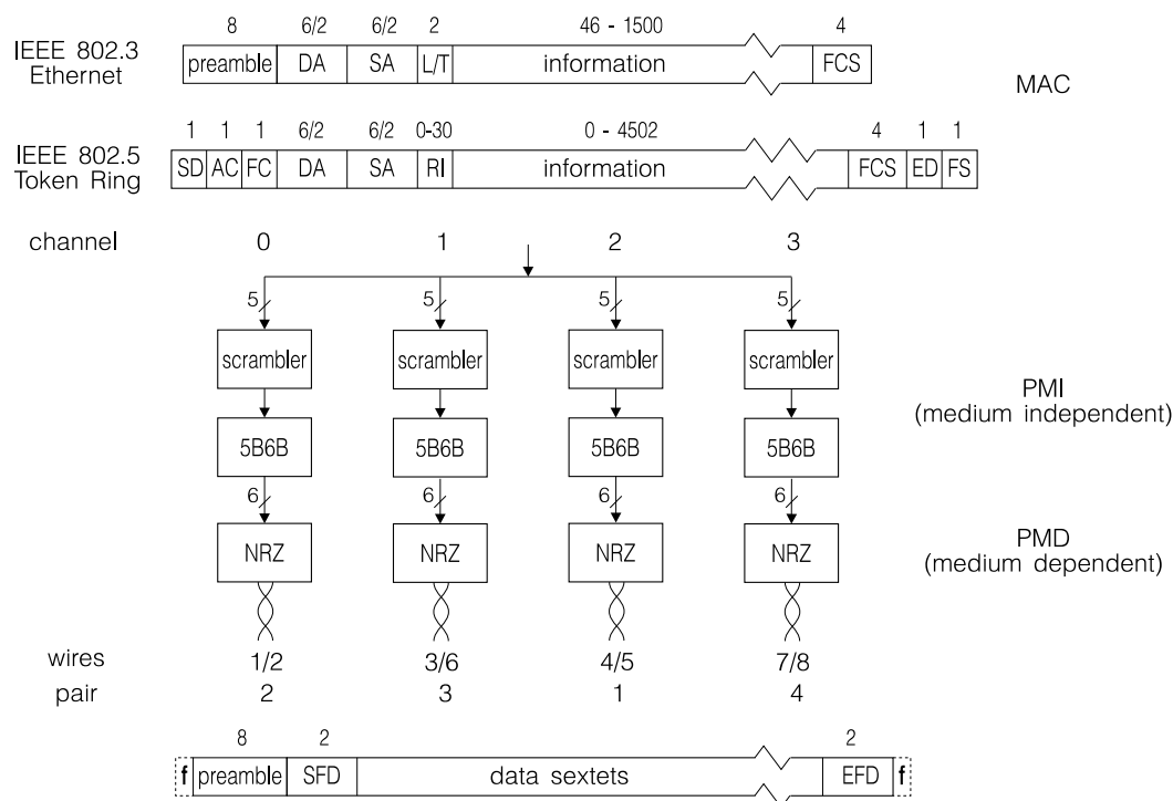
Obrázek 10.2: Kódování a struktura rámců sítě 100VG-AnyLAN
