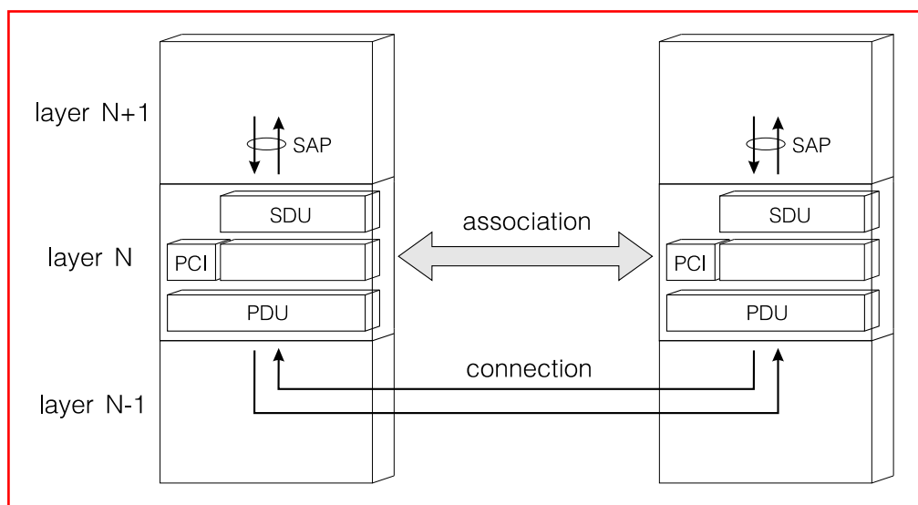
Obrázek 2.9: Vnitřní struktura vrstvy ISO OSI
