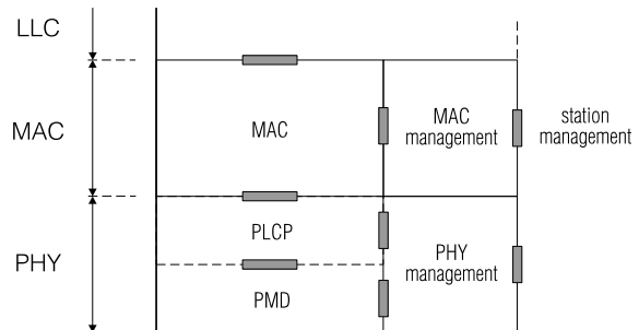
Obrázek 13.5: Architektura IEEE 802.11
