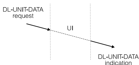
Obrázek 14.4: Nepotvrzovaný datagram
