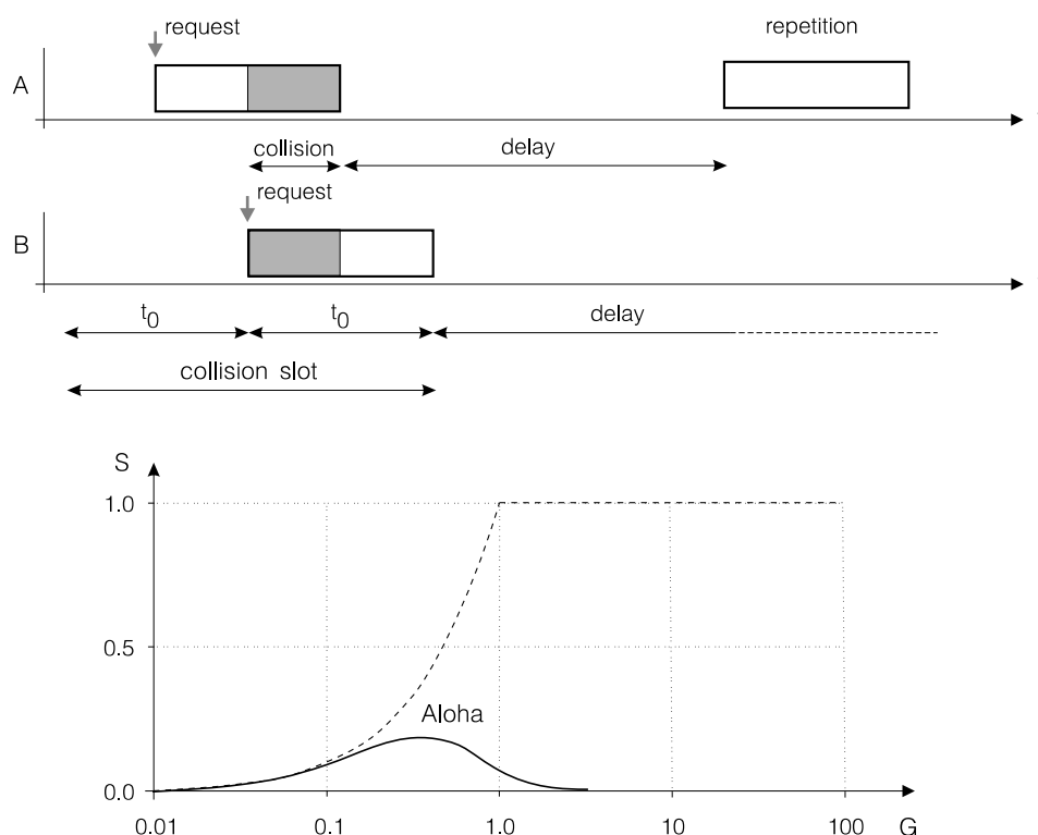
Obrázek 4.1: Prostá Aloha
