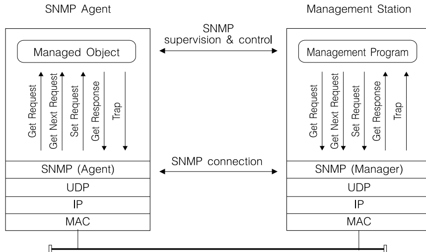
Obrázek 15.5: Komunikace SNMP
