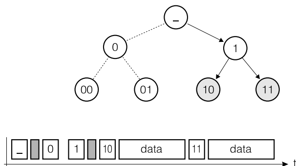
Obrázek 5.2: Binární vyhledávání
