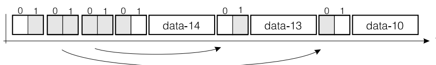
Obrázek 5.5: Binární vyhledávání
