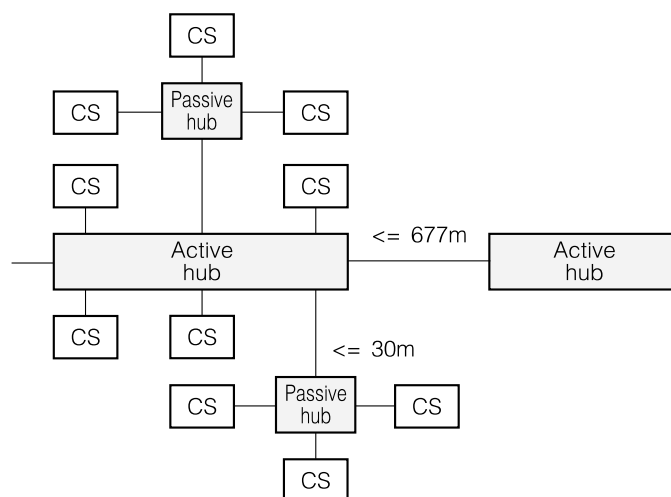
Obrázek 5.9: ARCNet – topologie
