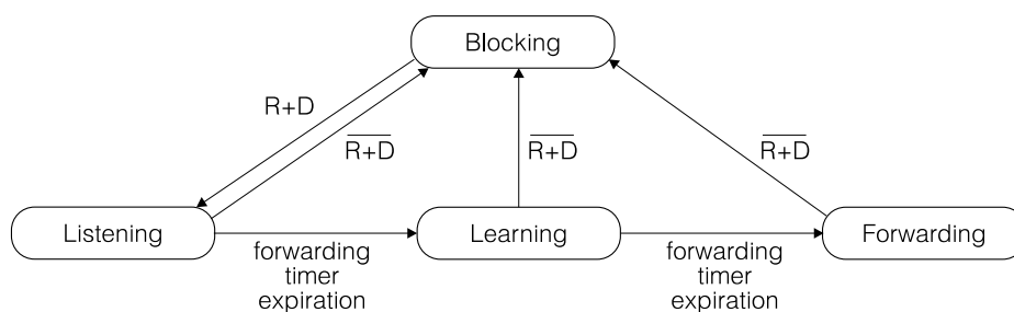
Obrázek 7.5: Stavový diagram transparentního mostu
