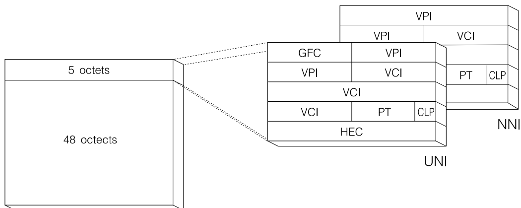
Obrázek 12.5: Buňka ATM
