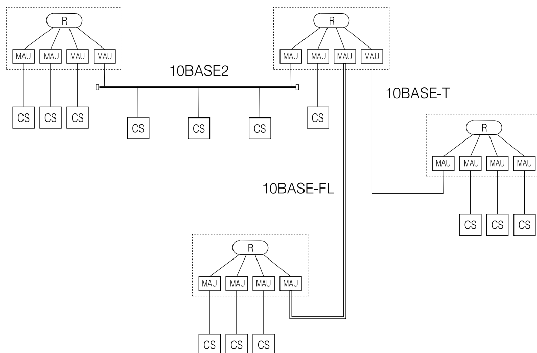
Obrázek 8.10: Struktura kombinovan0 sítě Ethernet
