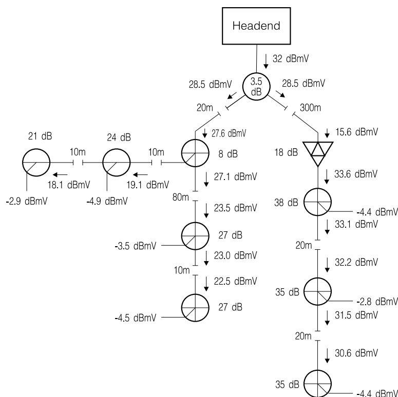
Obrázek 3.1: Širokopásmová síť
