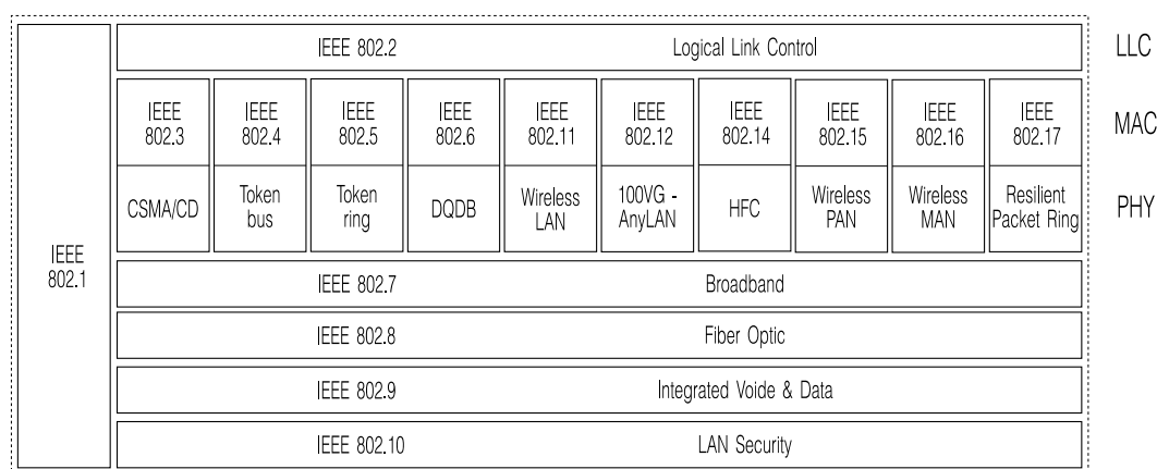
Obrázek 2.12: Technologie IEEE 802
