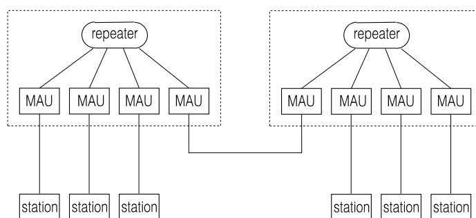
Obrázek 8.9: Struktura sítě 10BASE-T
