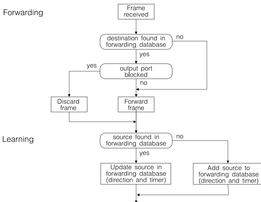
Obrázek 7.3: Činnost transparentního mostu
