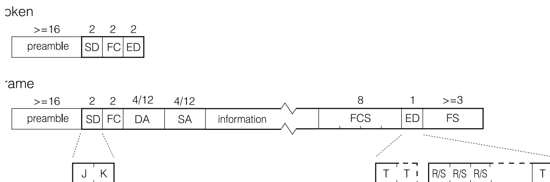
Obrázek 6.12: Formát rámce
