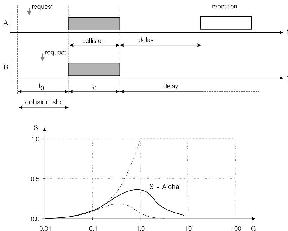
Obrázek 4.2: Taktovaná Aloha
