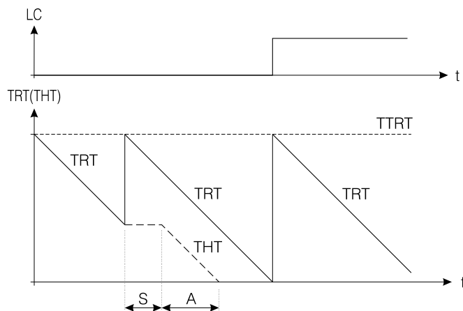
Obrázek 6.13: Přidělování kapacity
