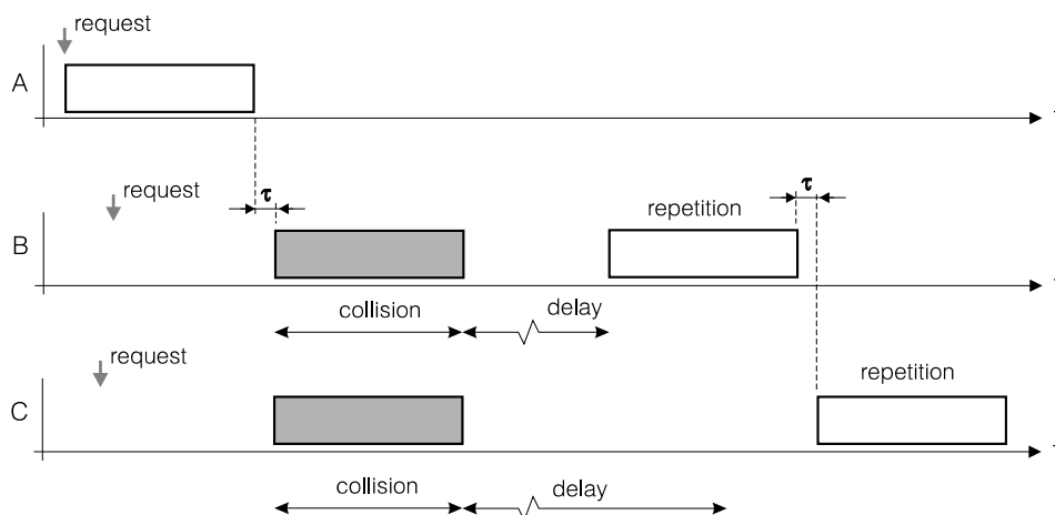
Obrázek 4.4: Naléhající CSMA
