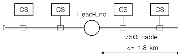
Obrázek 8.7: Technologie 10BROAD36
