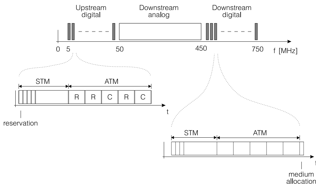
Obrázek 3.4: Rozdělení kmitočtového pásma sítě IEEE 802.14 Hybrid-Fibre-Coax System
