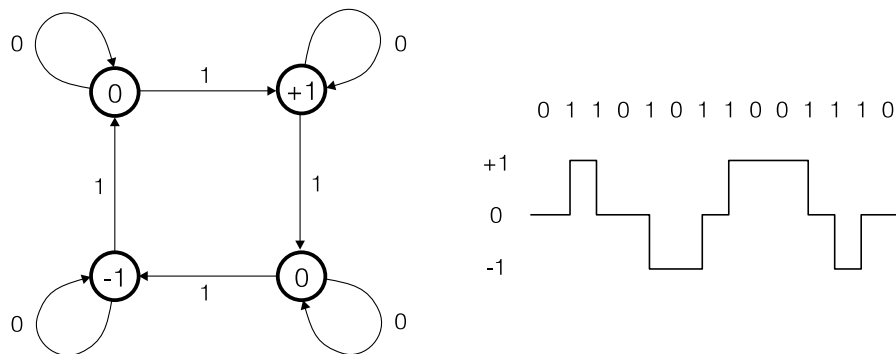
Obrázek 8.16: Kódování MLT-3
