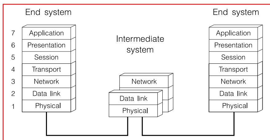
Obrázek 2.8: Architektura vrstev ISO OSI
