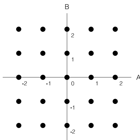
Obrázek 8.31: Kódování PAM-5
