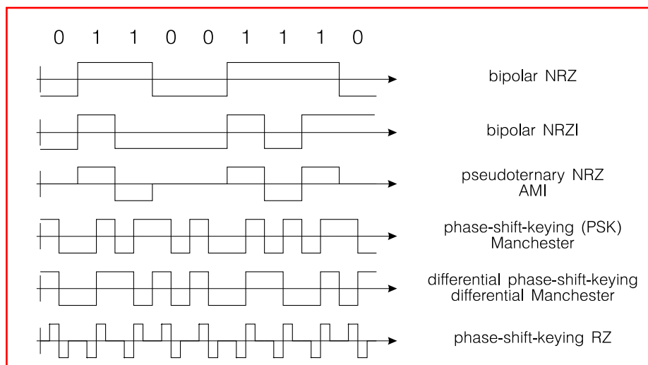
Obrázek 2.5: Kódování datového signálu v lokálních sítích
