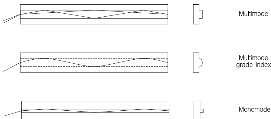
Obrázek 2.3: šíření signálu v optickém vlákne
