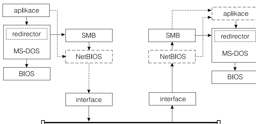
Obrázek 16.1: Struktura síťového rozšíření operačního systému MS-DOS MS-Net
