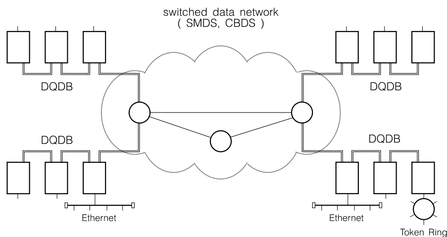
Obrázek 11.1: DQDB – Architektura metropolitní sítě s rohraním DQDB
